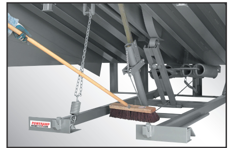
CleanSweep Frame permite un acceso despejado al área del pozo.
